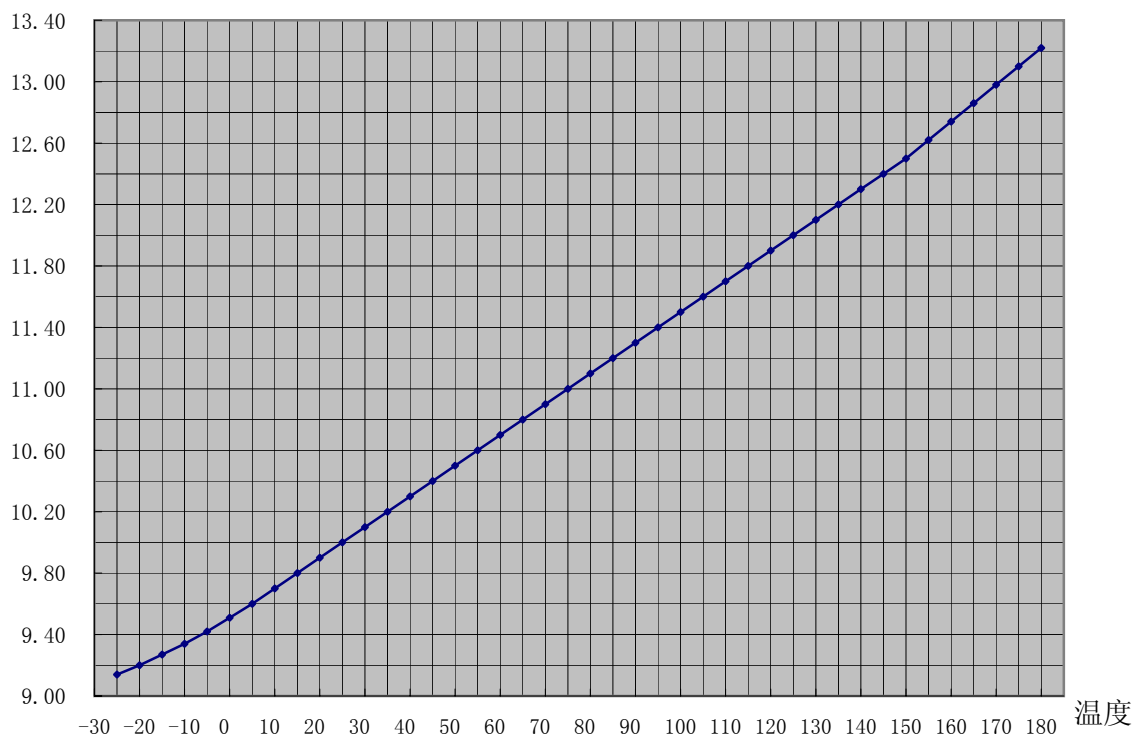
温度—阻值曲线图
